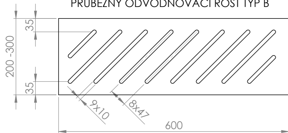
PRŮBĚŽNÝ ODVODŇOVACÍ ROŠT TYP B
