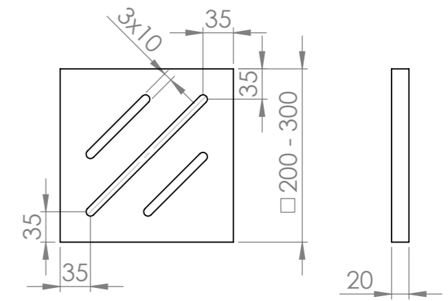
ROHOVÝ PRVEK ANG.
