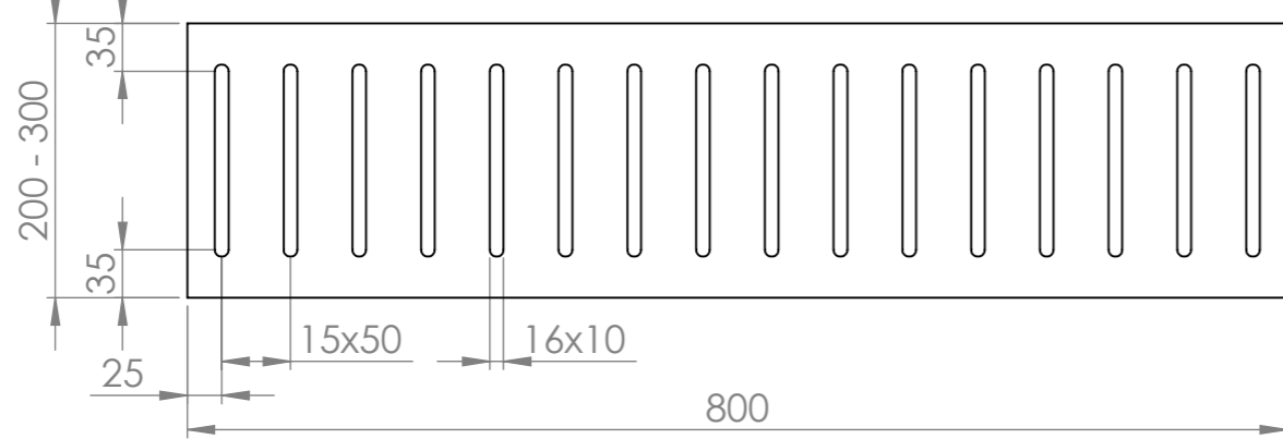
PRŮBĚŽNÝ ODVODŇOVACÍ ROŠT TYP A
