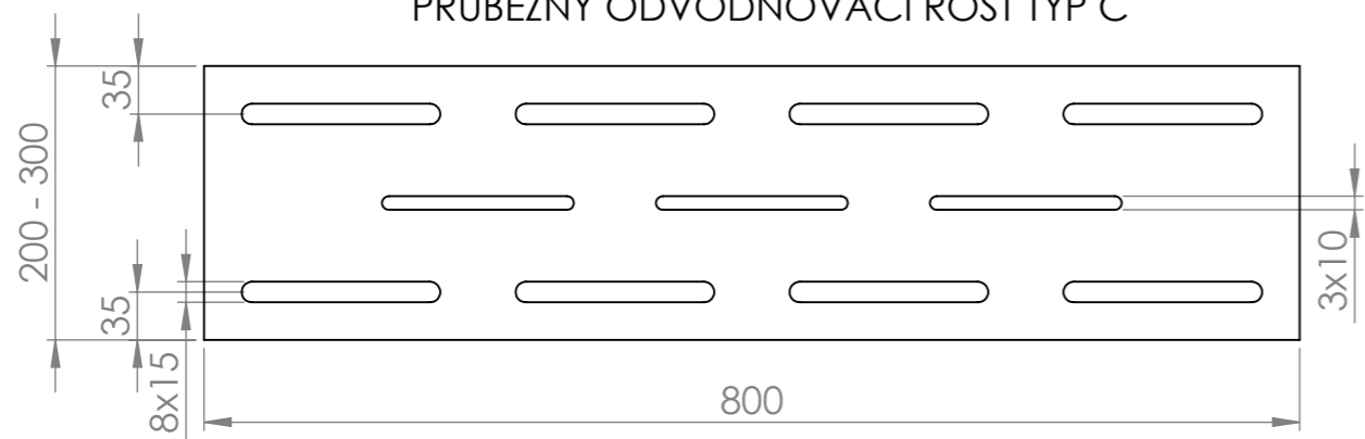
PRŮBĚŽNÝ ODVODŇOVACÍ ROŠT TYP C
