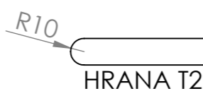
TYPY ZALEŠTĚNÝCH HRAN (DETAIL X) 1:4
