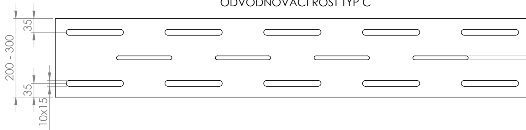
ODVODŇOVACÍ ROŠT TYP C
