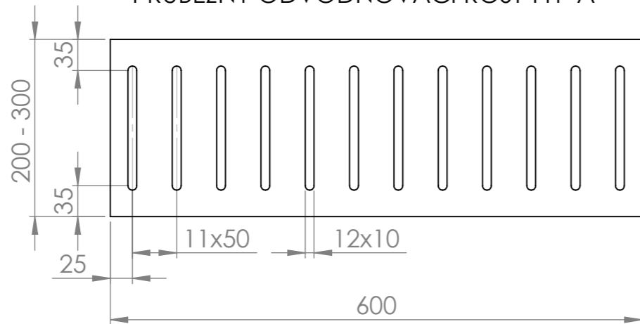
PRŮBĚŽNÝ ODVODŇOVACÍ ROŠT TYP A
