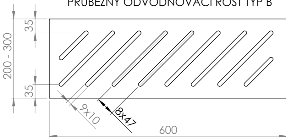
PRŮBĚŽNÝ ODVODŇOVACÍ ROŠT TYP B
