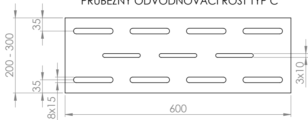
PRŮBĚŽNÝ ODVODŇOVACÍ ROŠT TYP C
