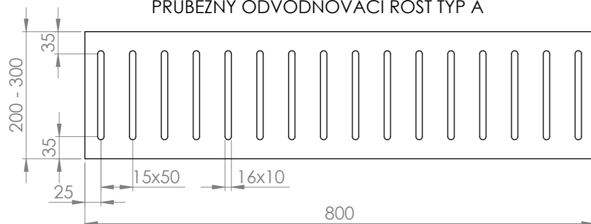
PRŮBĚŽNÝ ODVODŇOVACÍ ROŠT TYP A
