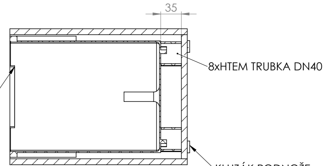
ŘEZ B-B
