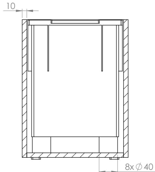
ŘEZ B-B
